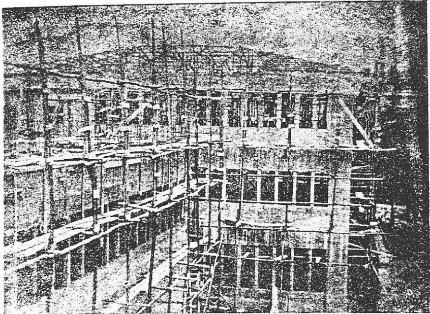
አዲሱ ፡ የመኝታ ፡ ቤት ፡ ሕንፃ ፡ ስሠራ ፡ The New Dormitory Building under Construction.
